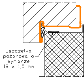
Rys. 7b Uszczelka ppoż. w drzwiach LF561C
