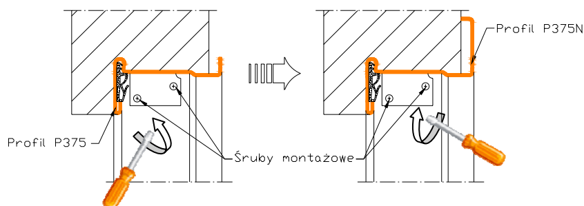
Rys. 1d Profil kierunkowy P375N
