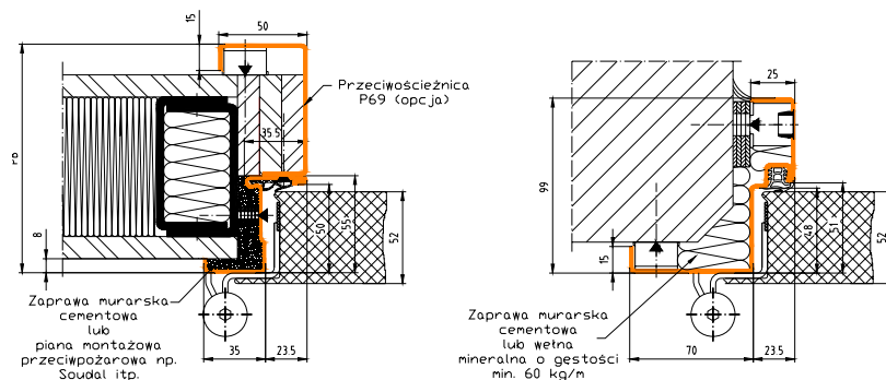
Rys. 3b Alternatywny sposób montażu ościeżnicy P375D / P375+69D oraz P25D
