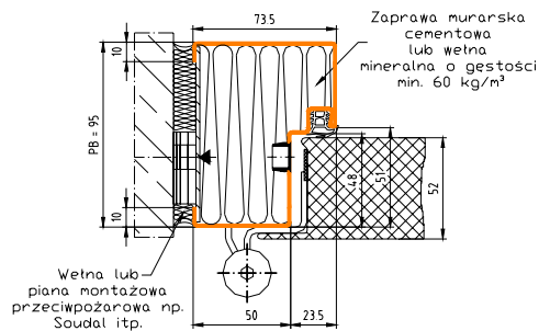
Rys. 3c Ościeżnica blokowa P34D
