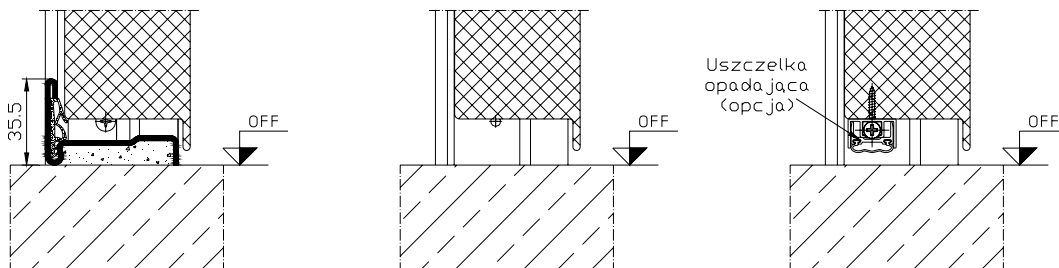
Rys. 1a Drzwi z progiem
