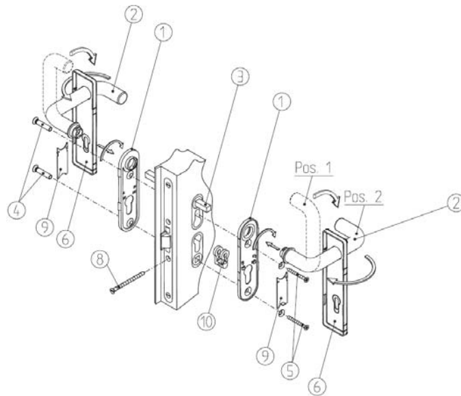
Rys. 4 Okucie z krótkim sztyldem (standard dostawy)
