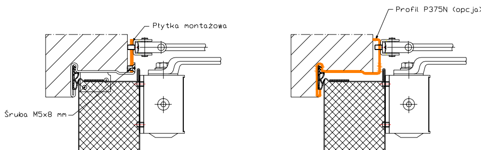
Rys. 6 Montaż samozamykacza w drzwiach LF531E / LF561C
