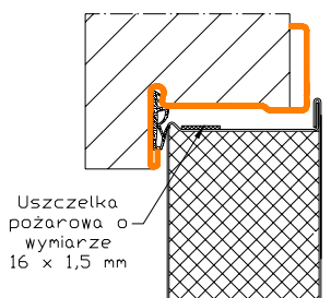
Rys. 7a Uszczelka ppoż. w drzwiach LF531E
