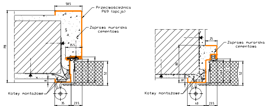
Rys. 3a Montaż ościeżnicy P375M / P375+69M oraz P25M poprzez rozgięcie kotew
