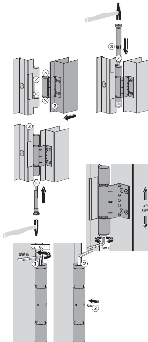
Rys. 5 Instrukcja montażu zawiasów
