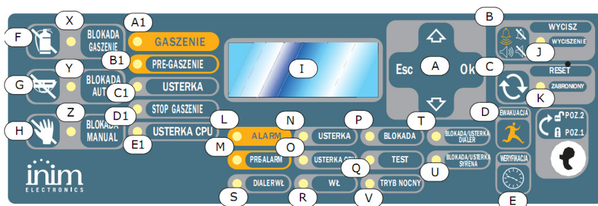
Rysunek 1 – Płyta czołowa centrali
